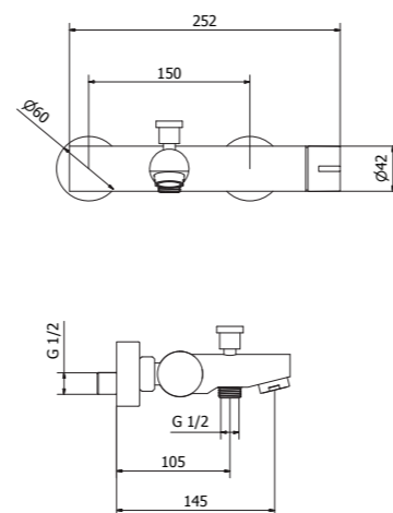
2H540 Bath mixer
