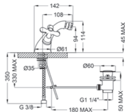
6247E One hole bidet mixer
